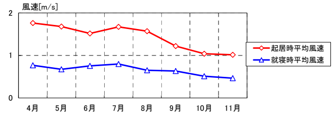
図2 平均風速
