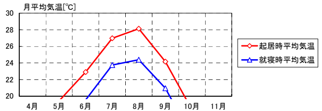
図3 平均気温
